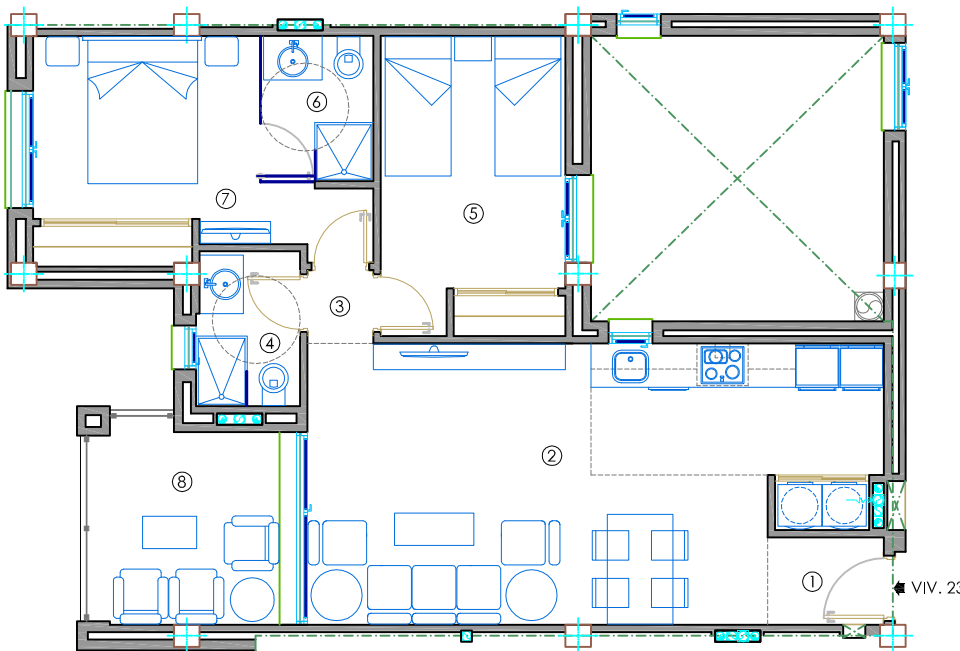
PLANTA DE MOBILIARIO
